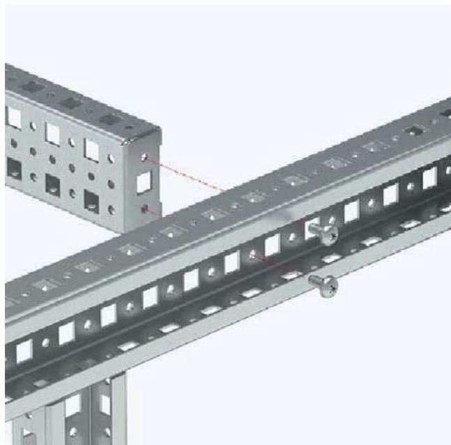
Соединение профилей с помощью болтов M5x10
